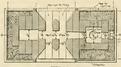
SECTION A-B.
